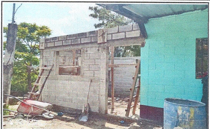
Foto 2: Area frontal, donde se esta realizando el mejoramiento las paredes y la estructura tipo portico para la cocina, piso y polleton como tambien ventanas y puertas.
